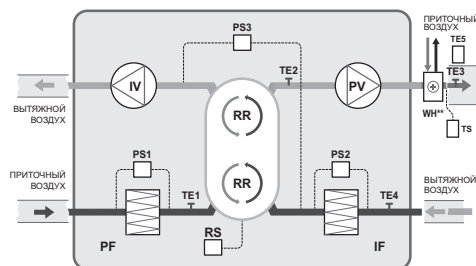
ZPVR-N-PW-EC, Вид снизу (со стороны обслуживания)
