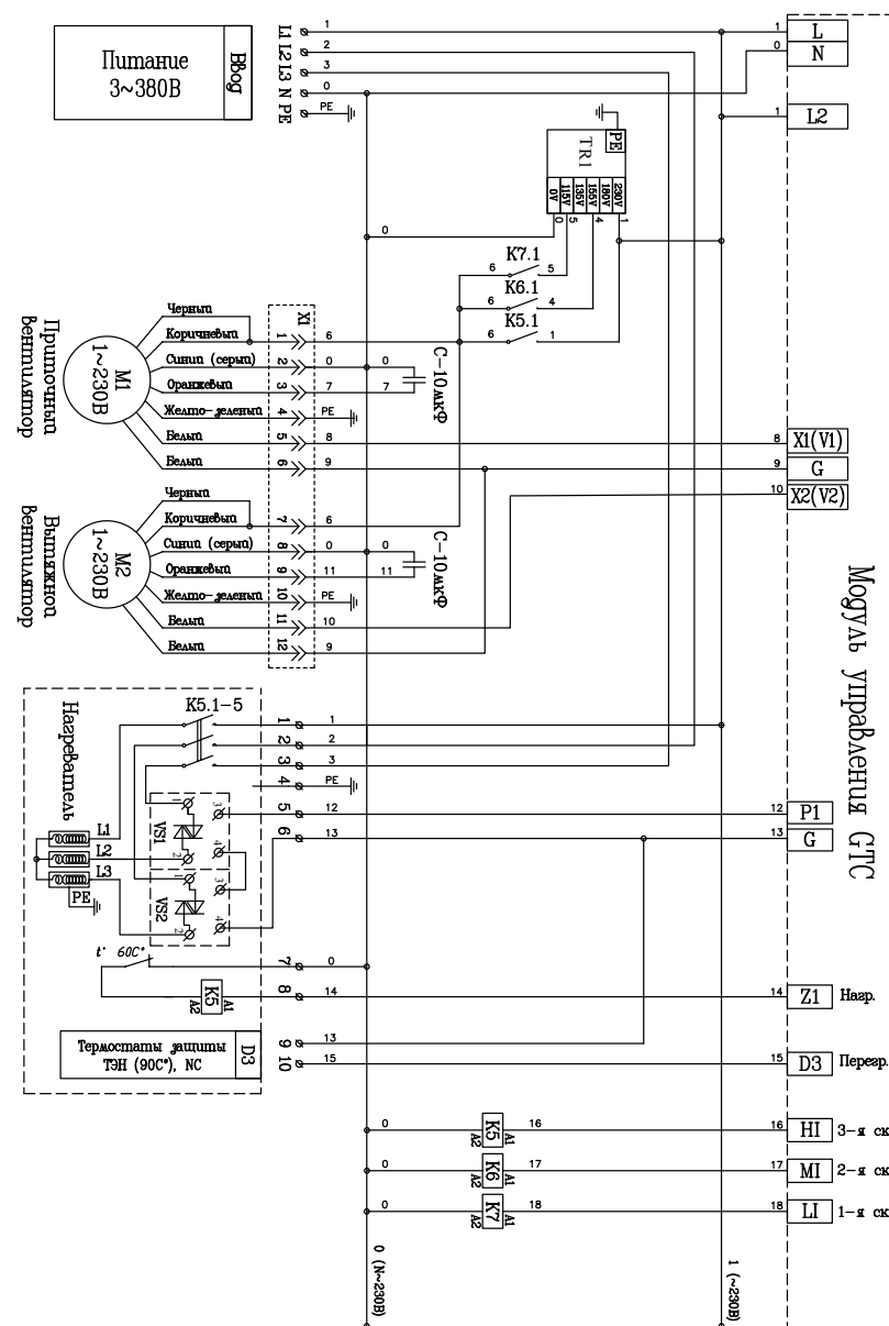
Схема ZPVP 2000 VE
