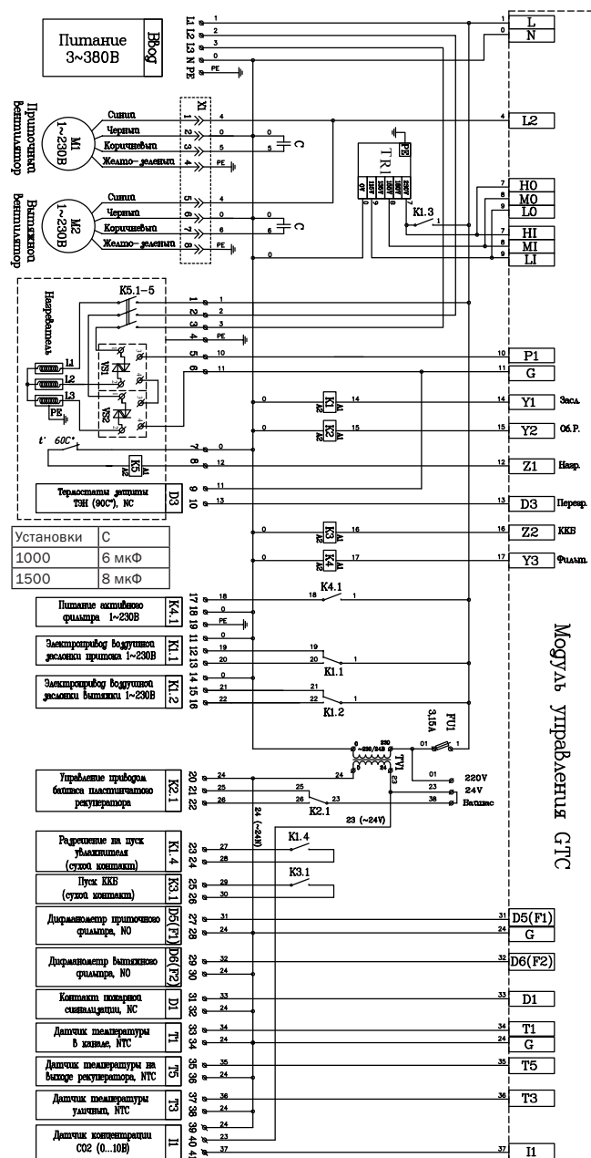
Схема ZPVP 1000 VE, ZPVP 1500 VE
