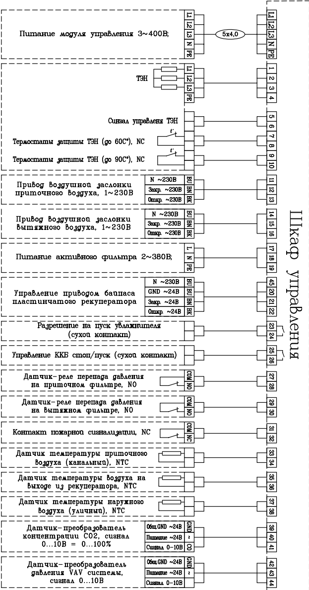
Схемы подключения ZPVP 1400 PE EC, ZPVP 2200 PE EC
