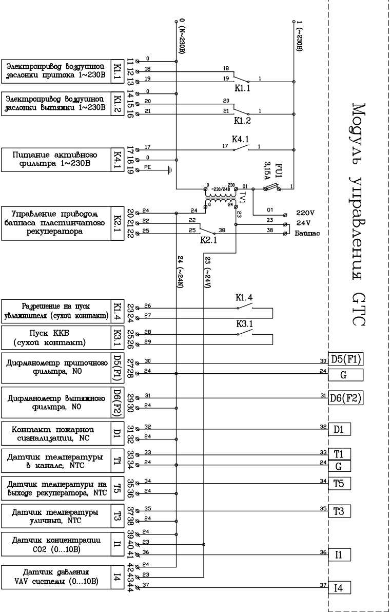
Схемы подключения ZPVP 1400 PE EC, ZPVP 2200 PE EC
