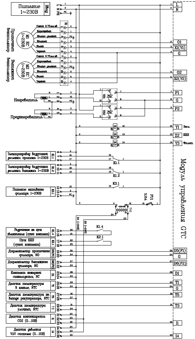
Схема подключения ZPVP 450 PE EC, ZPVP 850 PE EC
