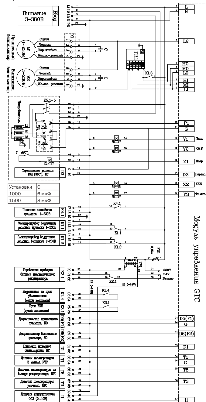
Схема ZPVP 1000 HE, ZPVP 1500 HE
