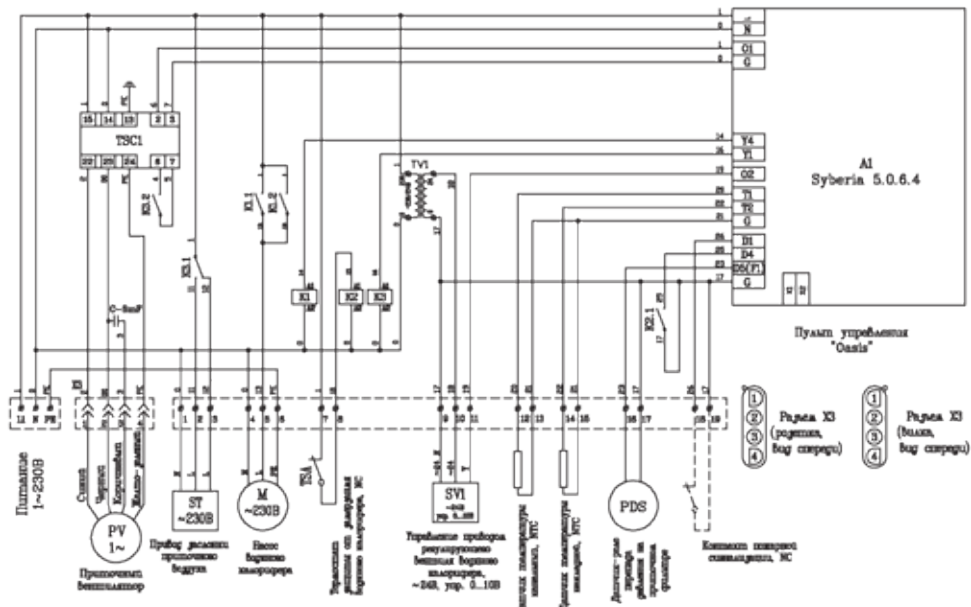
Схема для установок с водяным нагревателем
