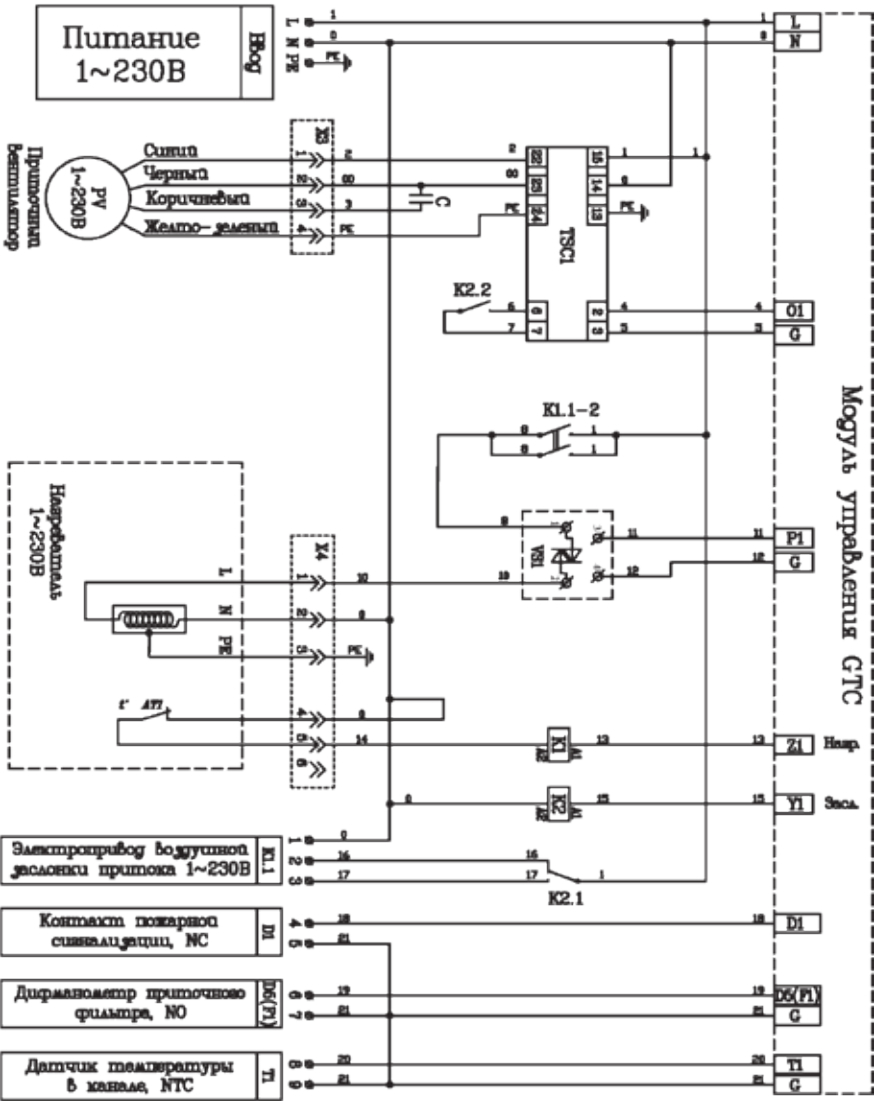
Схема для установок с электрическим нагревателем 1 фазным
