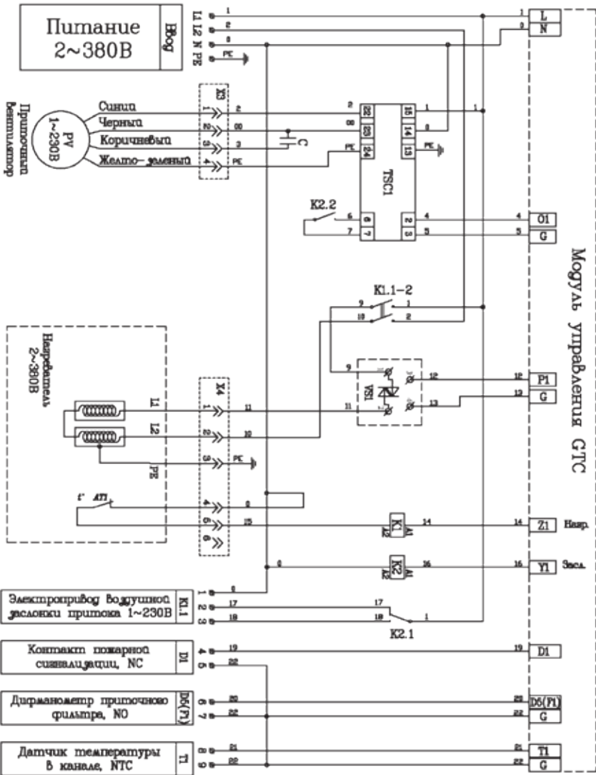
Схема для установок с электрическим нагревателем 2-х фазным
