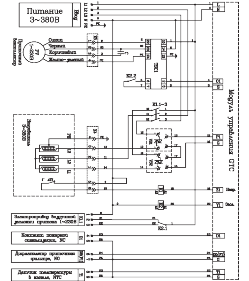
Схема для установок с электрическим нагревателем 3-х фазным
