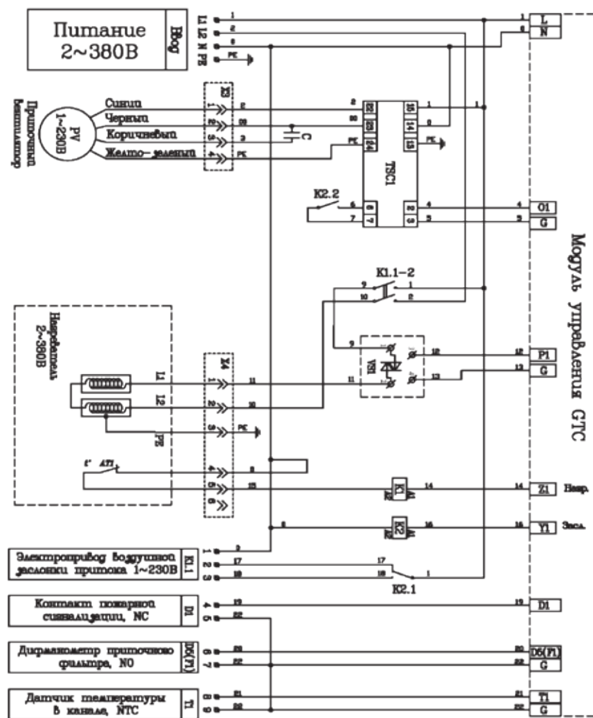
Схема для установок с электрическим нагревателем 2-х фазным
