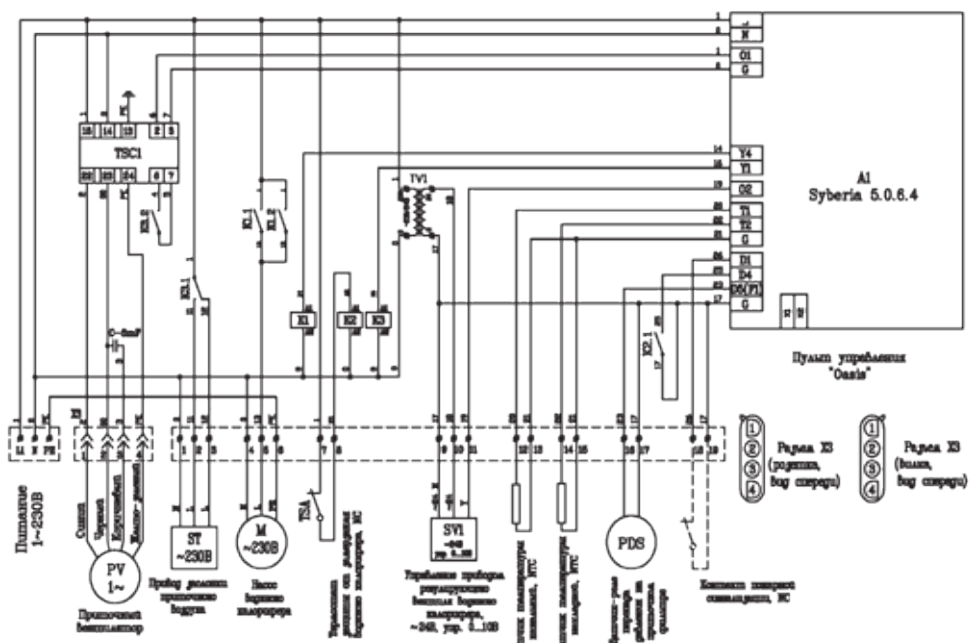
Схема для установок с водяным нагревателем
