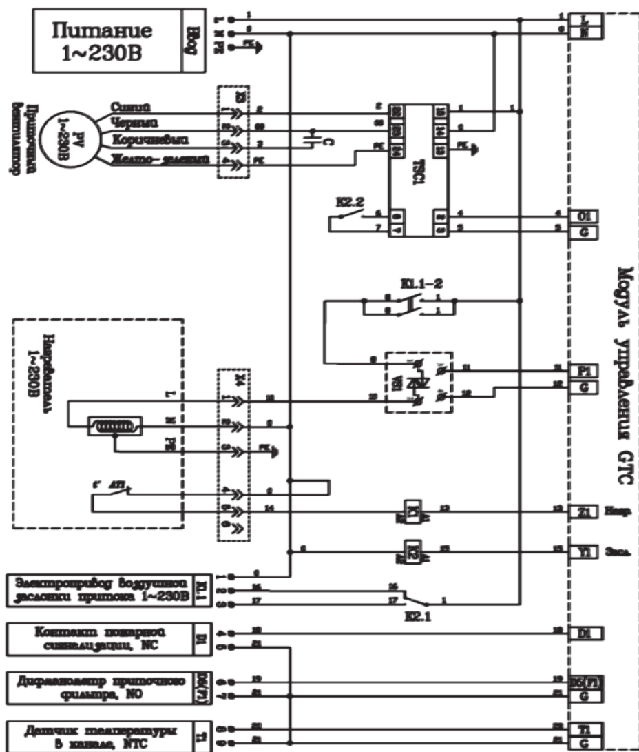
Схема для установок с электрическим нагревателем 1 фазным
