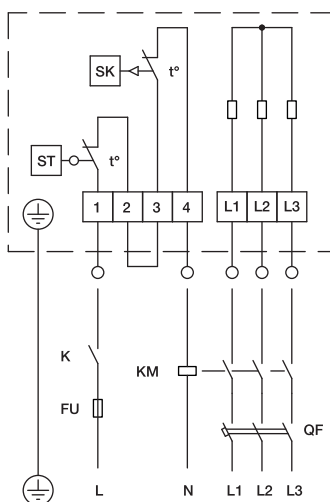
Схема 4 (400 В, 3 фазы)
