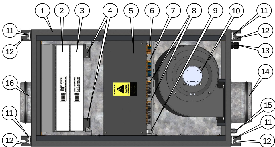
Рисунок 1. Конструкция. Установлены кассетные воздушные фильтры М5 и Е11
