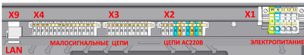
Рис. 2 Расположение клемм
