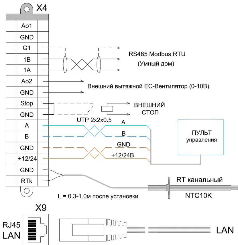
Рис. 8 Схема подключения оборудования. Малосигнальные цепи
