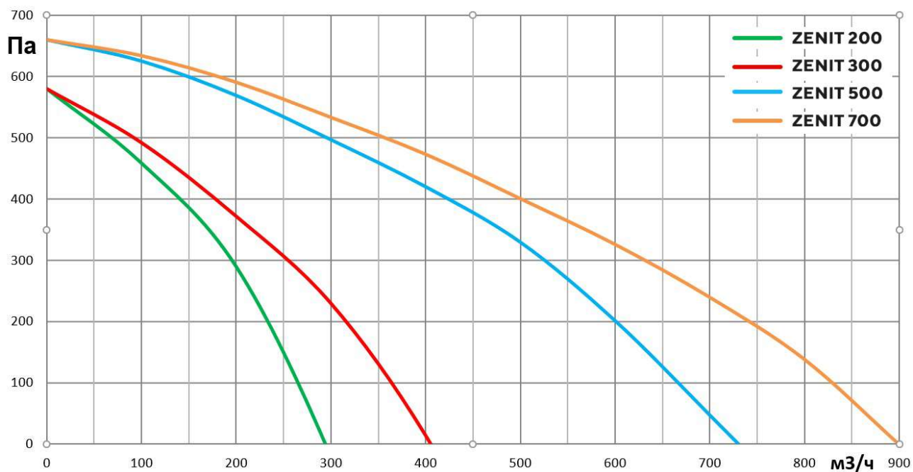
Графики статического давления оборудования
