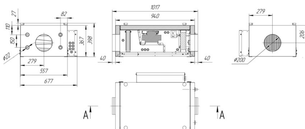
Рис.1б Габариты и присоединительные размеры Torvex SF02 M
