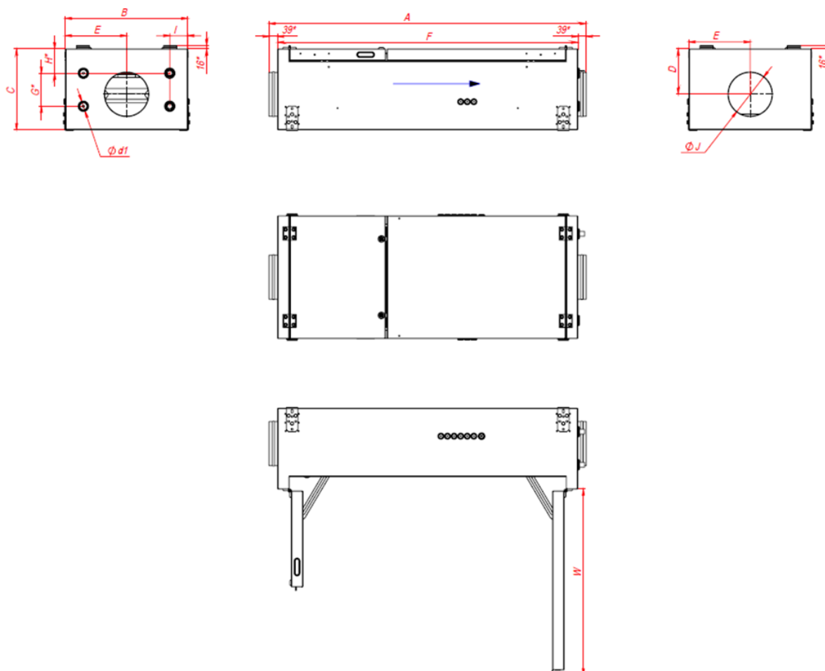
Рис.1а Габариты и присоединительные размеры Torvex SF02
