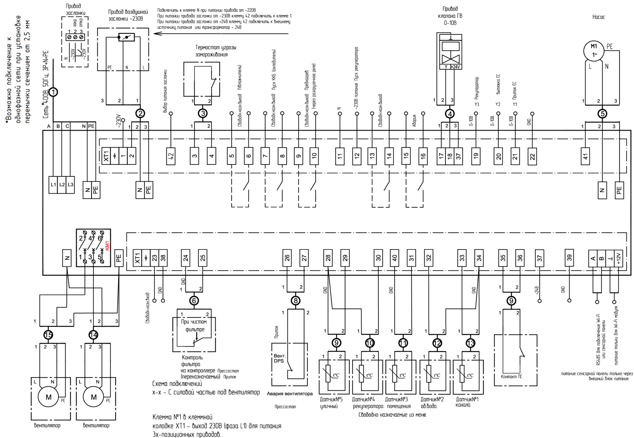
Электрическая схема (внешнее подключение) Torvex FR 03 HW
