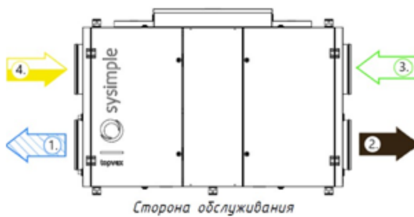
Рис.2 Расположение потоков воздуха в зависимости от левого и правого исполнения агрегата Torvex FR
