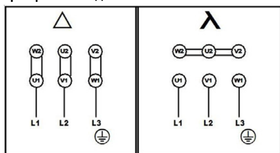
Двигатель Gamak
