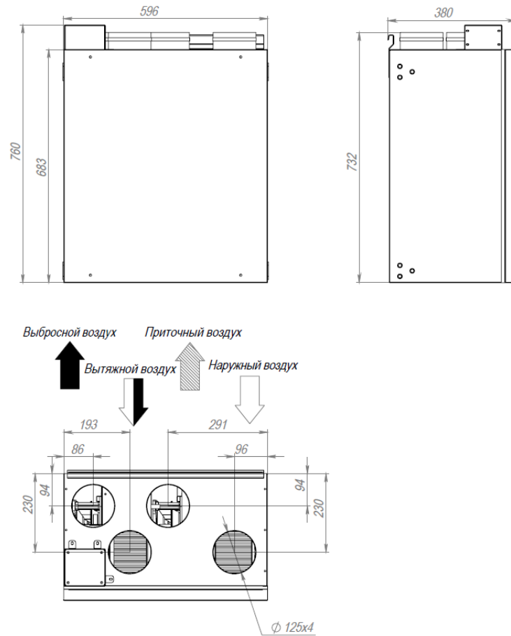
Рис.1.1 - Габариты и присоединительные размеры SAVE VTR 150
