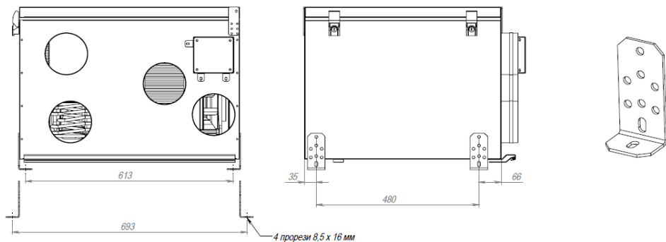
Рис.2.3 - Габариты монтажных кронштейнов для подвесного исполнения SAVE VTR 325 (опция)
