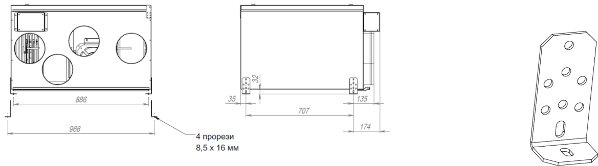
Рис.2.2 - Габариты монтажных кронштейнов для подвесного исполнения SAVE VTR 500 (опция)
