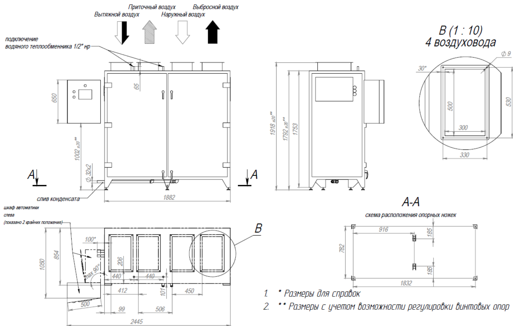
Рис.2 Конфигурация Geniox TX25 с установленными гибкими вставками для подключения воздухопроводов вверх
