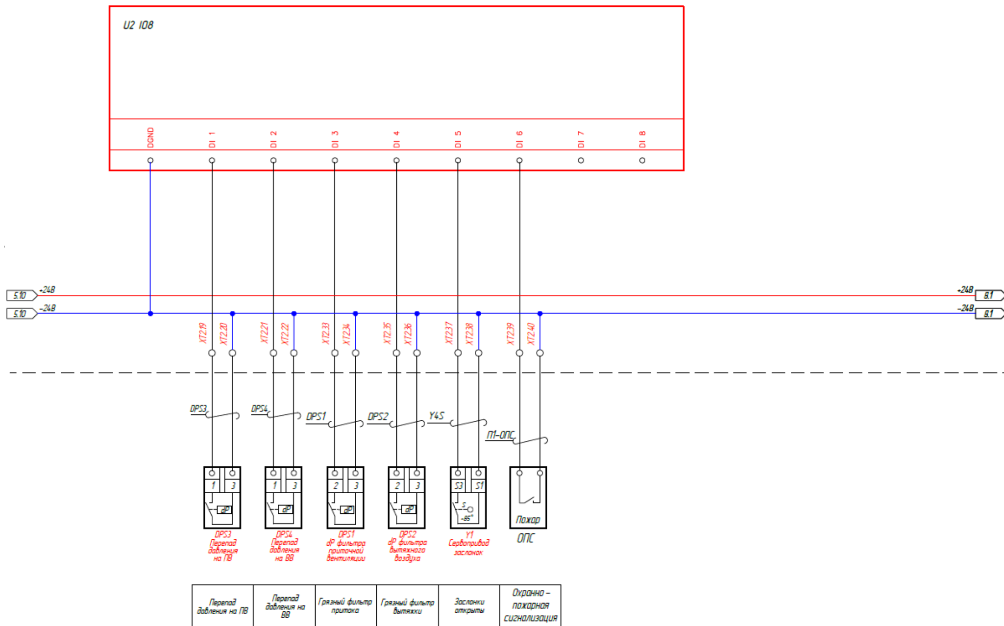
Рис.16(8) Схема электрическая принципиальная Geniox TX 25
