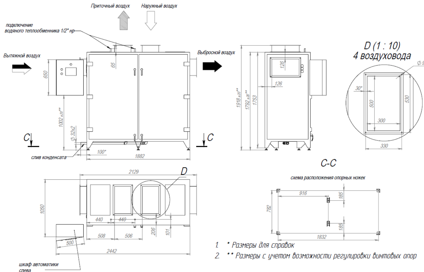
Рис.1 Конфигурация Geniox TX25 с установленными гибкими вставками для подключения воздуховодов вверх и вбок
