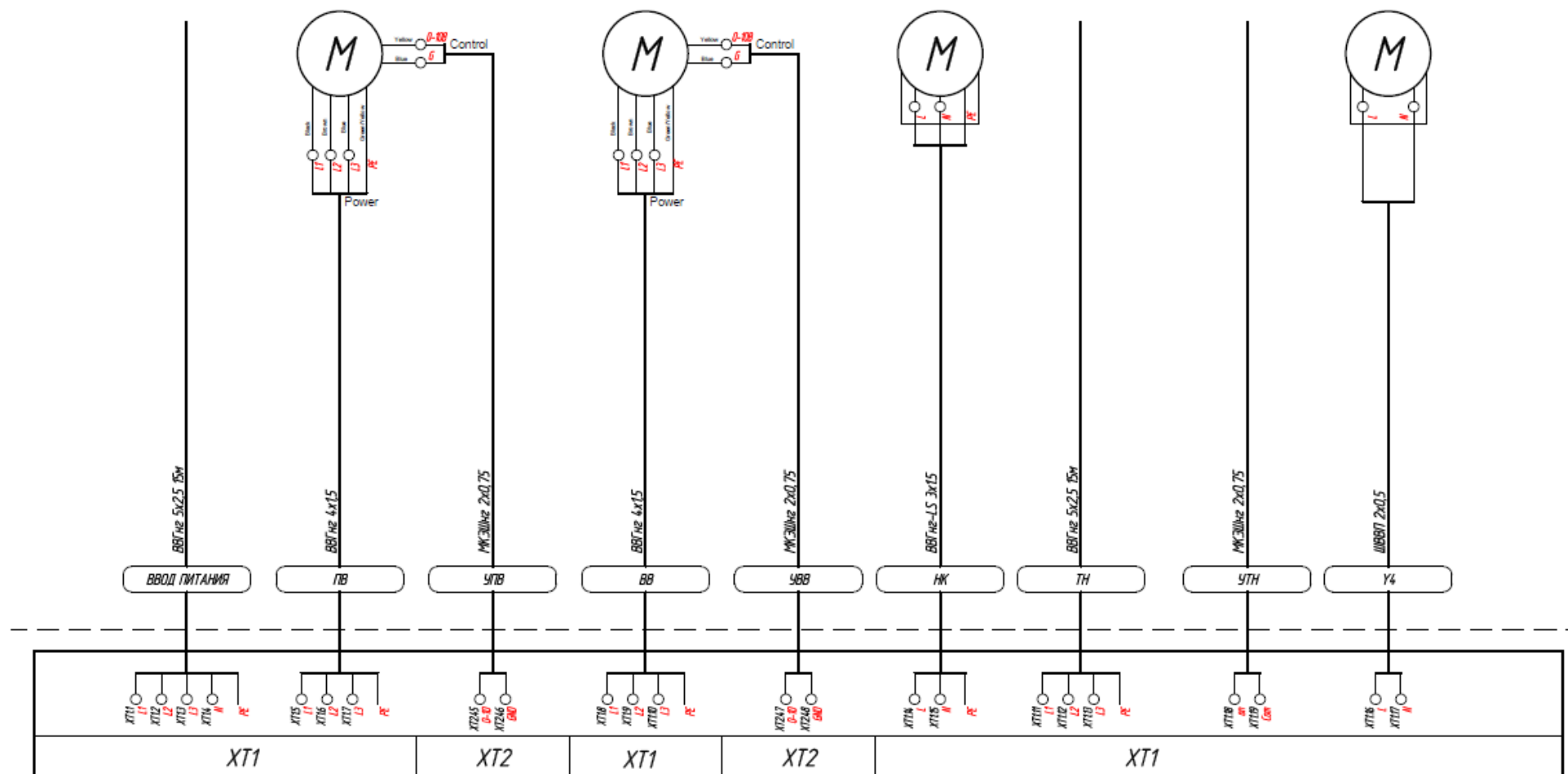
Рис.11(10) Схема электрическая принципиальная Geniox Pool
