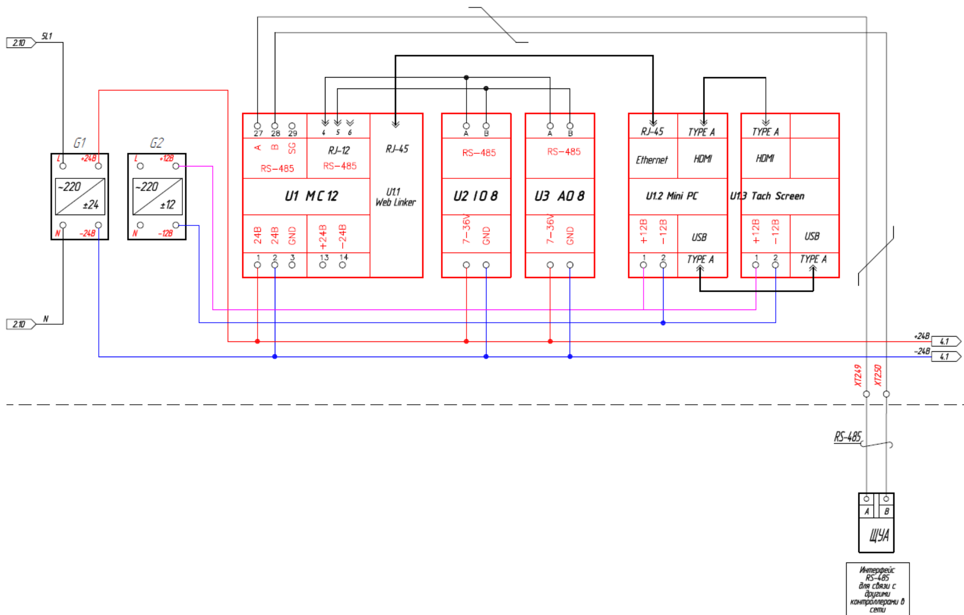
Рис.11(3) Схема электрическая принципиальная Geniox Pool
