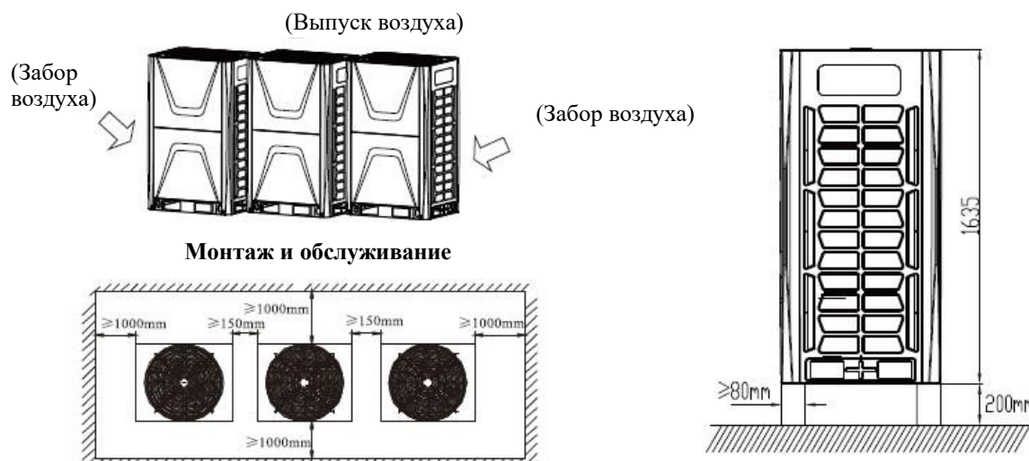
Пространство для монтажа наружного блока
