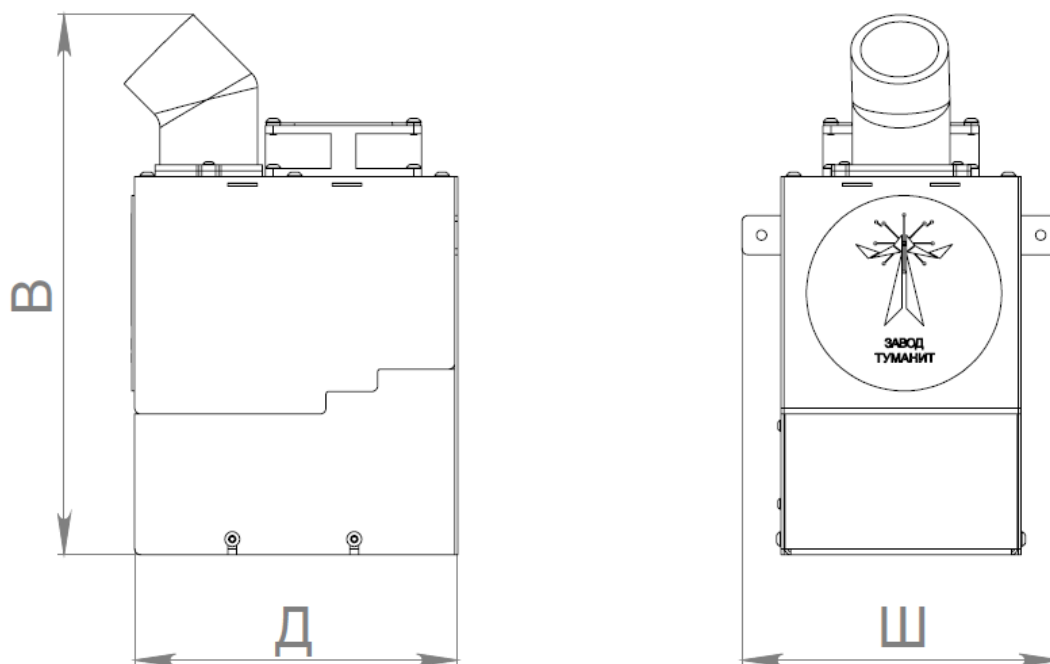
Рис.1 Модуль генерации
