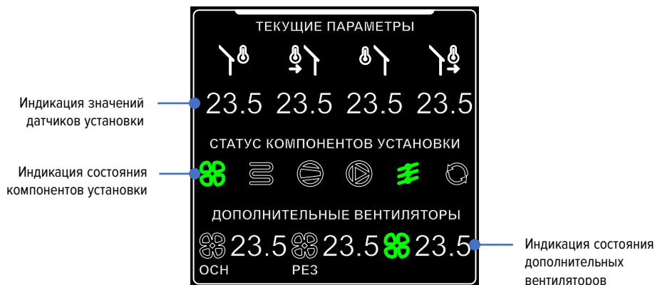
Рис. 17. Информация о состоянии компонентов установки
