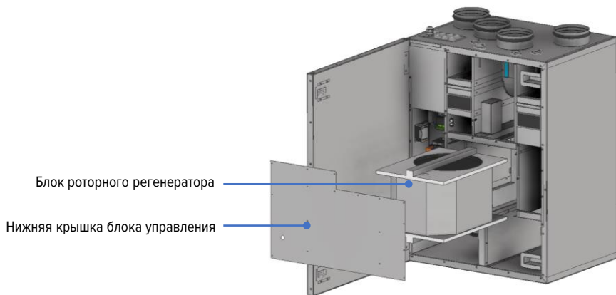
Рис. 28. Обслуживание роторного регенератора
