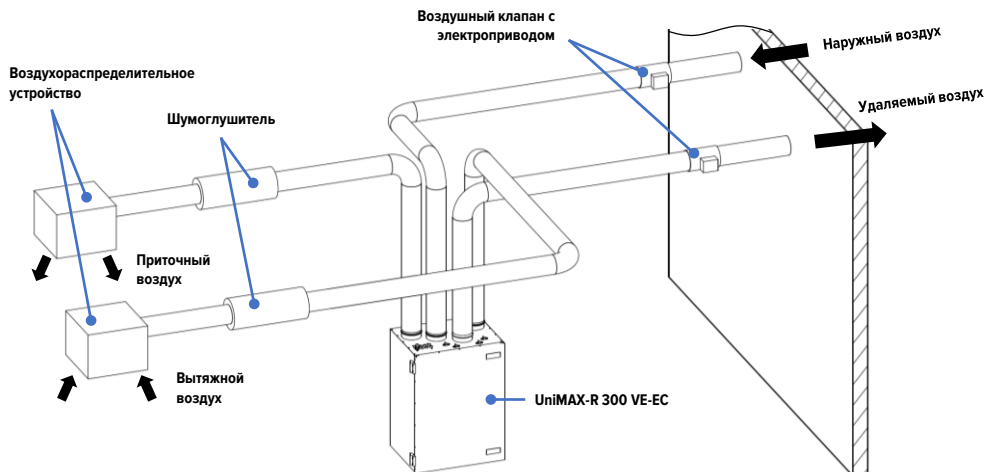
Рис. 9. Монтажная схема
