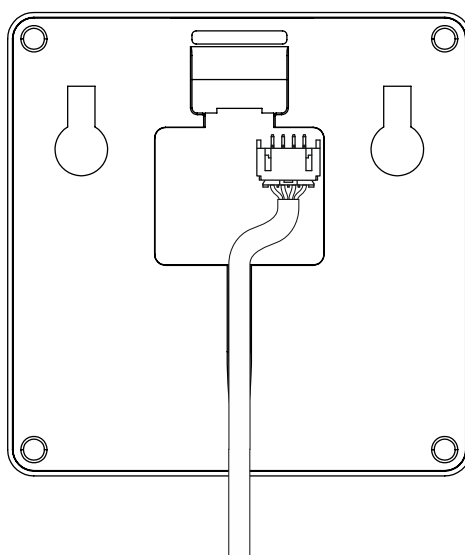
Размещение кабеля после подключения
