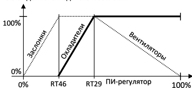
Охлаждение: охладитель и заслонки
