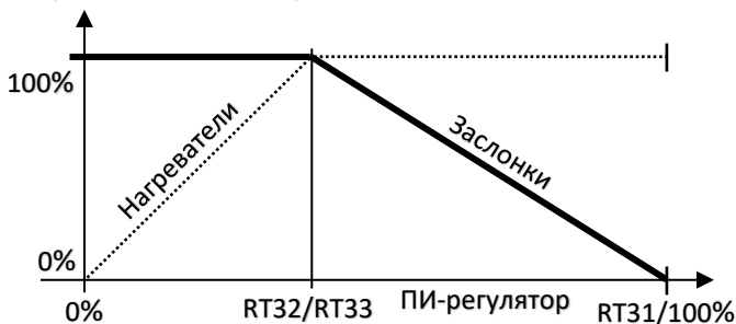
Нагрев: заслонки и нагреватели
