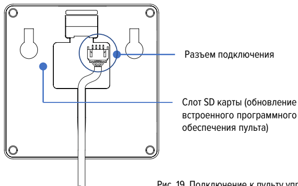
Рис. 19. Подключение к пульту управления
