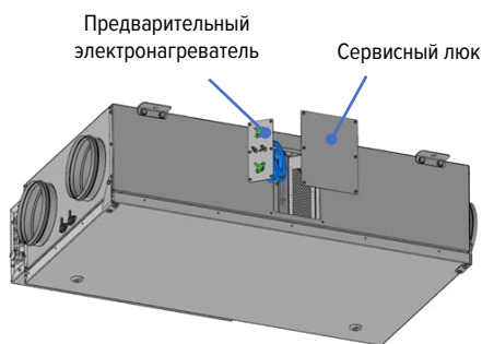
Рис. 40. Обслуживание предварительного электронагревателя
