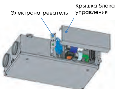
Рис. 34. Обслуживание электронагревателя
