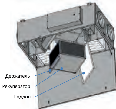
Рис. 32. Обслуживание рекуператора на UniMAX-P 1000 CE-A
