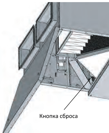
Рис. 28. UniMAX-P 1500 CE-A
