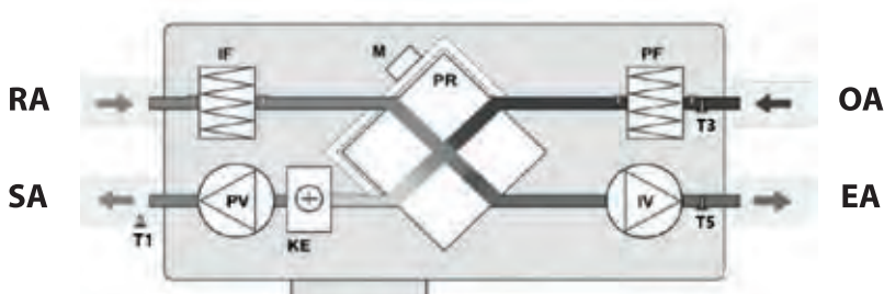
Рис. 6. Принципиальная схема UniMAX-P 1000/1500 CE-A
