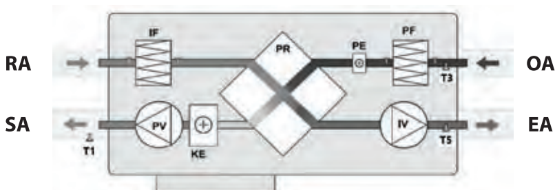
Рис. 5. Принципиальная схема UniMAX-P 450/800 CE-A
