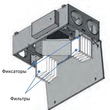
Рис. 30. Обслуживание вентилятора
