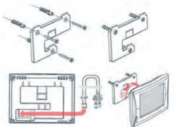
Рис. 18. Монтаж пульта управления
