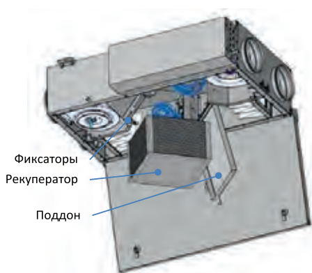
Рис. 31. Обслуживание рекуператора на UniMAX-P 450/800 CE-A
