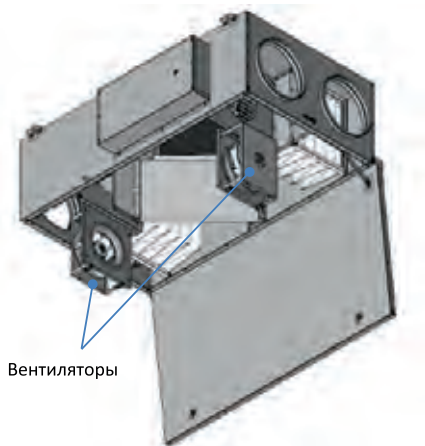
Рис. 33. Обслуживание вентилятора
