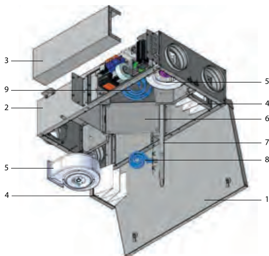
Рис. 1. Состав установки UniMAX-P 450 CE-A
