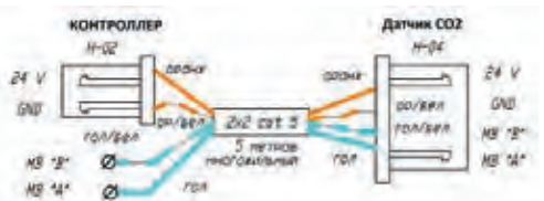
Рис. 23. Кабель для подключения внешнего датчика CO2
