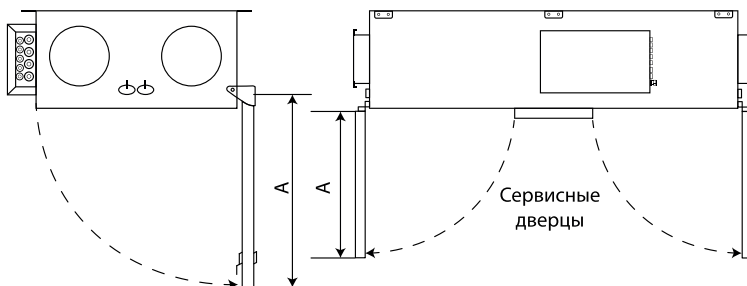
Рис. 9. UniMAX-P 450/800/1000 CE-A
