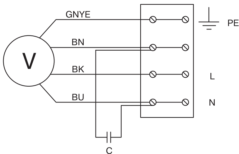
Схема №1 (1-230 В)
