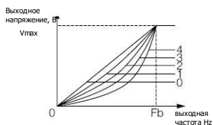
Vmax — максимальное выходное напряжение, Fb — максимальная выходная частота
