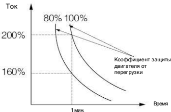
Рис. FA-1 Коэффициент защиты двигателя от перегрузки
