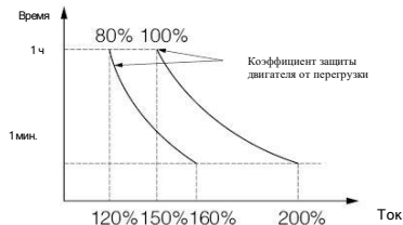
Рис. FA-2 Настройка коэффициента защиты двигателя от перегрузки
