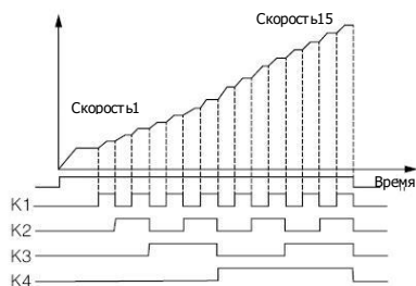
Рисунок F7-1 Многоскоростной режим работы 19: Выбор времени ускор./замедл. TT1 20: Выбор времени ускор./замедл. TT2 Путем выбора комбинации ON[вкл]/OFF[выкл.] данных функциональных клемм, можно выбрать максимум 4 вида времени ускор./замедл., как показано в следующей таблице:
