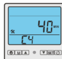
Параметры C4 Значение кода: Цикл размораживания Диапазон настройки: (20 мин ~ 90 мин) Согласие: 40 мин
