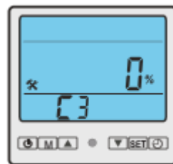
Параметры C3 Значение кода: ошибка датчика влажности. Согласие: 0 %.
