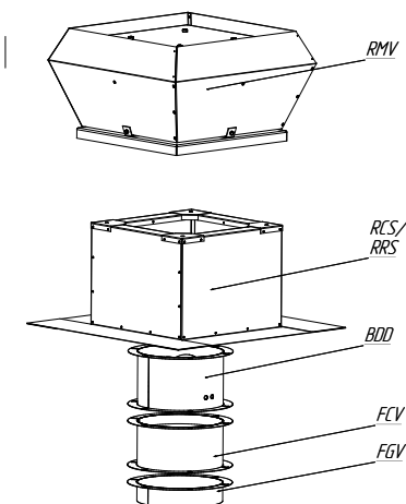
Монтаж вентилятора с коробом RCS, RRS (со встроенным шумоглушителем)
