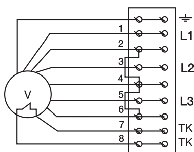
Схема №6 (400 В, 3 фазы)
