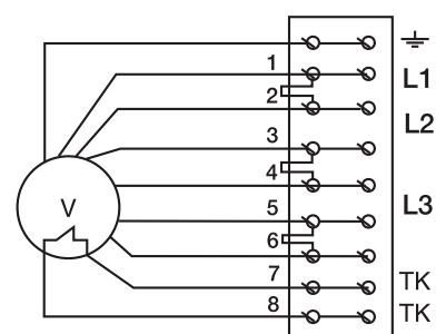
Схема №6 (400 В, 3 фазы)
