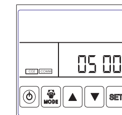
Рис. 32. Концентрация CO 2
