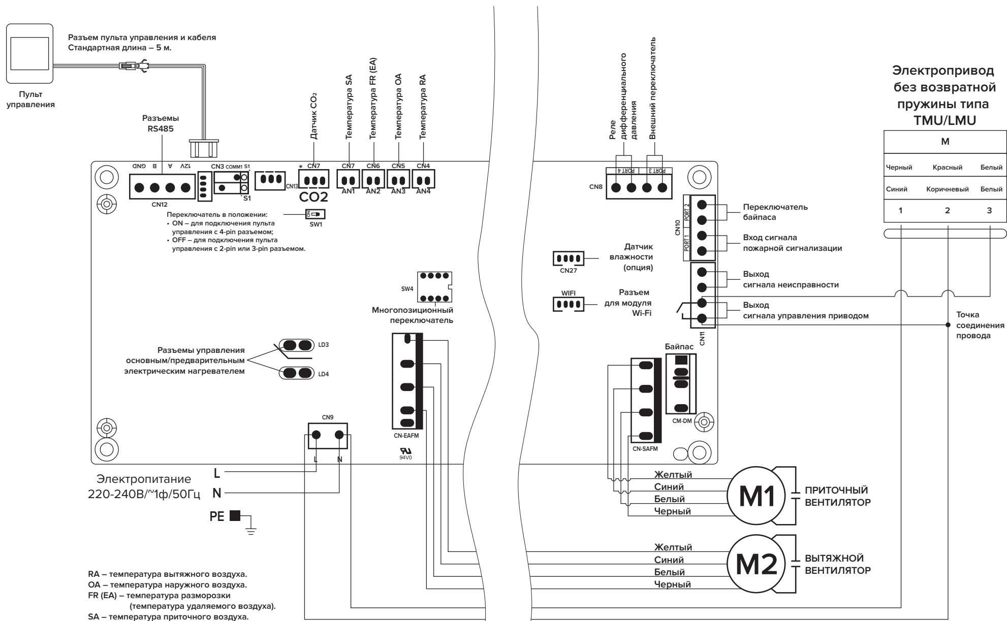
Рис. 15. Подключение электропривода без возвратной пружины
