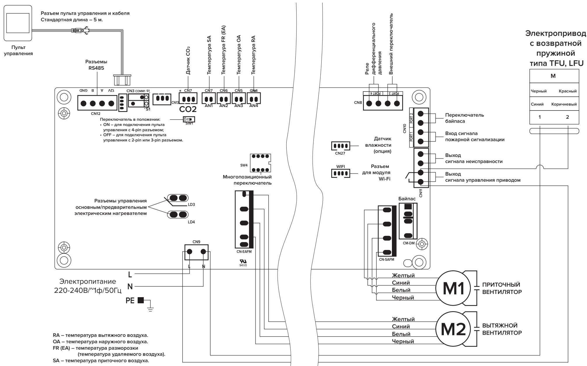
Рис. 16. Подключение электропривода с возвратной пружиной
