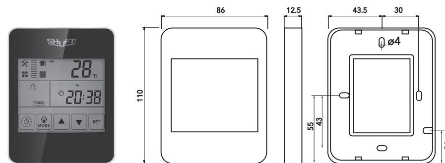
Рис. 20. Пульт управления SRC-TS
