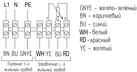
Схема подключения однофазного двигателя с установленным регулятором скорости
