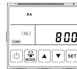
Концентрация CO 2
