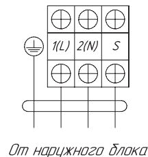
Клеммный терминал внутреннего блока
