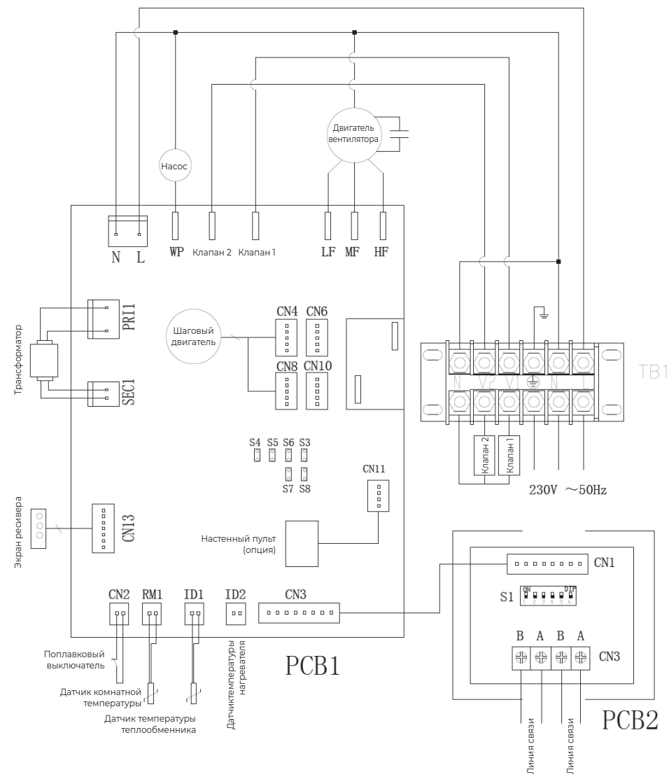
Схема подключения MACS-I-C_P4K
