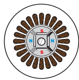
Центрированная обмотка
