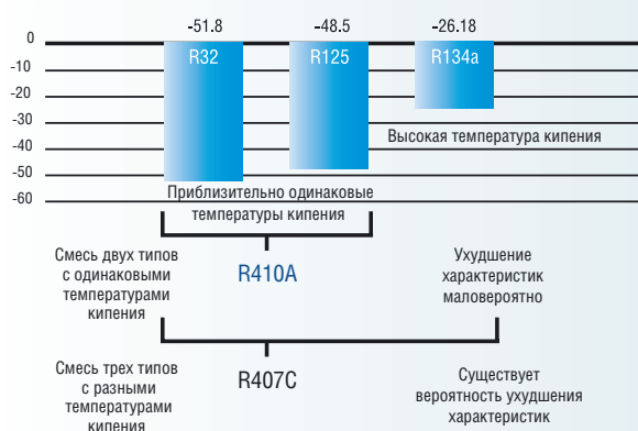
Сравнение температур кипения хладагента (жидкий и газообразный)
