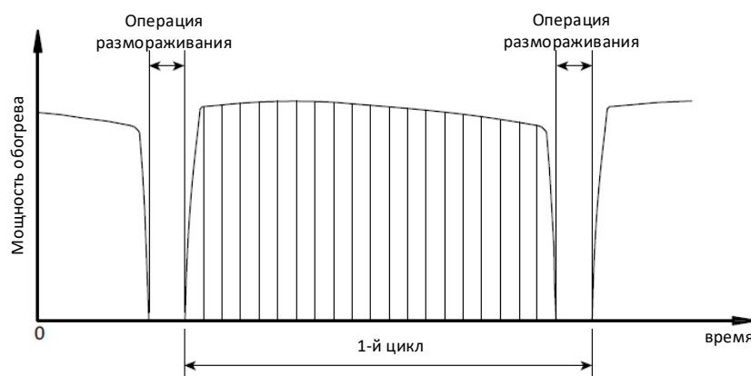
Рисунок 2-8.3. Цикл размораживания
