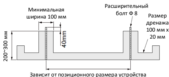
Рисунок 3-2.4. Типовой проект конструкции бетонного основания наружного блока (ед. изм.: мм)
