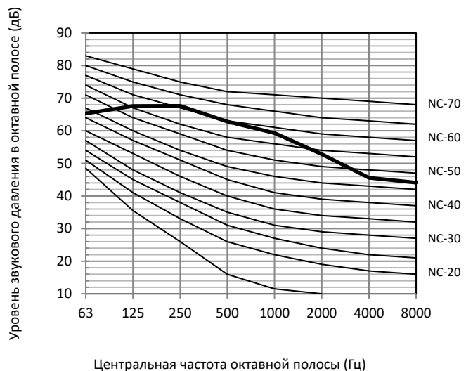
Рисунок 2-10.10. Уровень октавной полосы модели 24 л. с.
