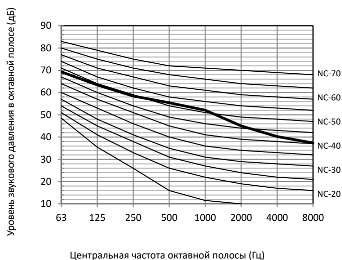
Рисунок 2-10.3. Уровень октавной полосы модели 10 л. с.
