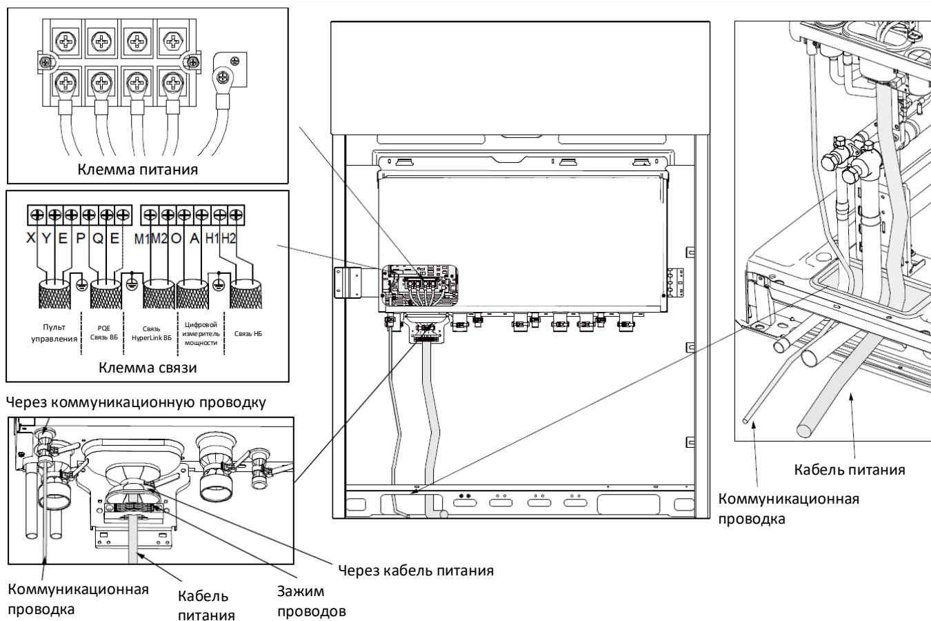
Рисунок 3-9.1. Схема электропроводки
