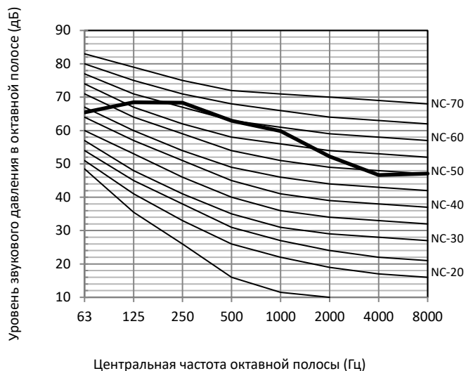
Рисунок 2-10.8. Уровень октавной полосы модели 20 л. с.
