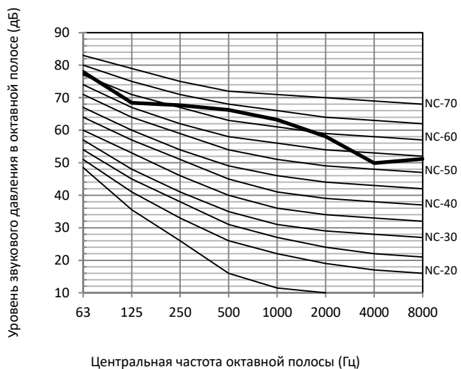
Рисунок 2-10.12. Уровень октавной полосы модели 28 л. с.
