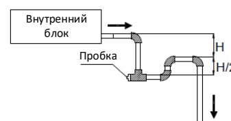
Рисунок 3-6.6. Сифоны дренажных трубопроводов
