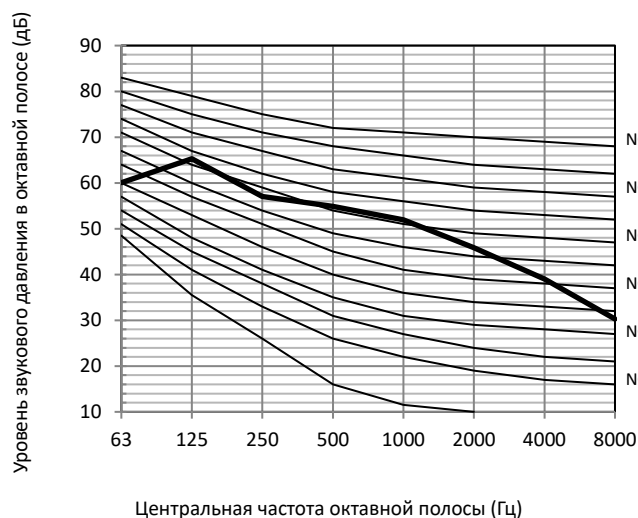
Рисунок 2-10.2. Уровень октавной полосы модели 8 л. с.
