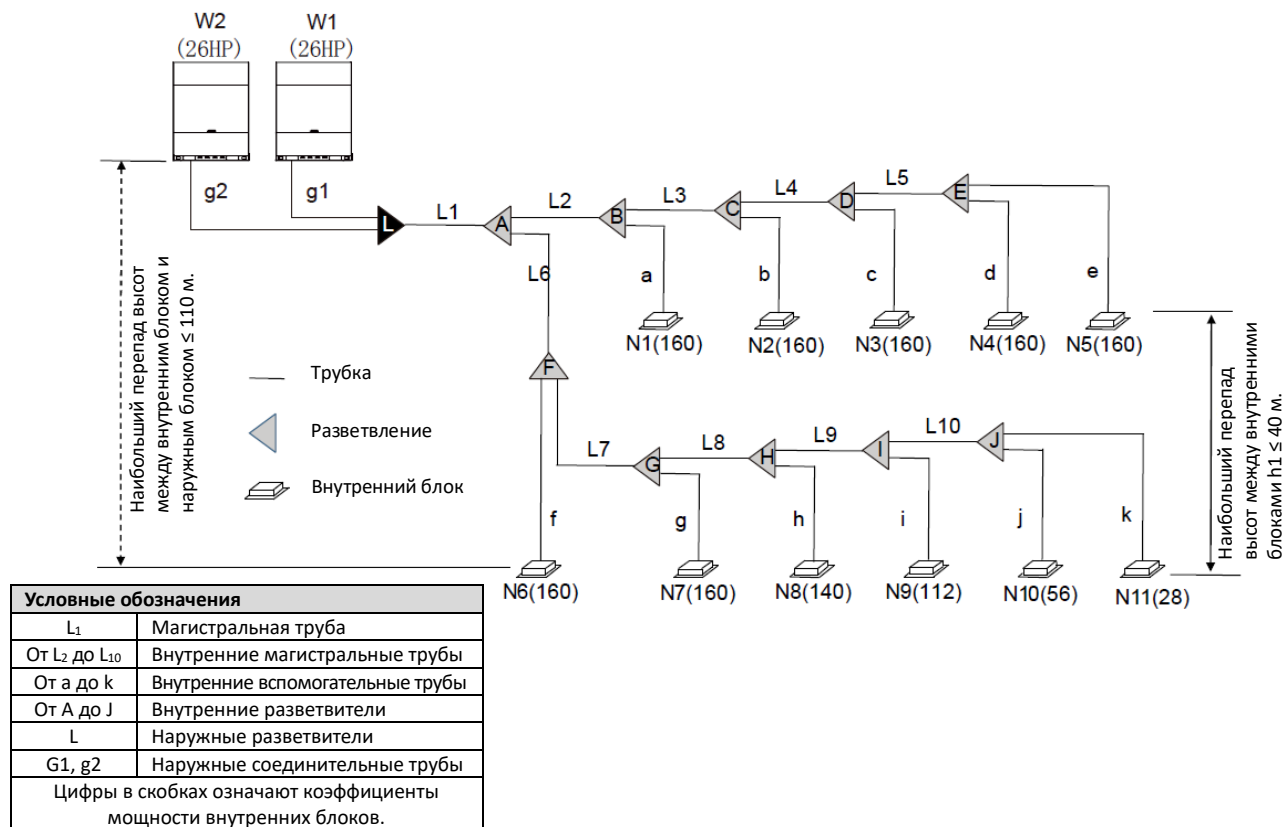
Рисунок 3-4.4. Пример выбора трубопровода хладагента
