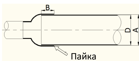
Рисунок 3-5.7. Перекрытие трубопроводов и зазор для паяных соединений
