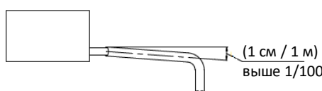
Рисунок 3-6.1. Требования к минимальному уклону дренажного трубопровода
