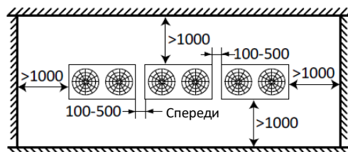
Рисунок 2-3.2. Однорядная установка (ед. изм.: мм)
