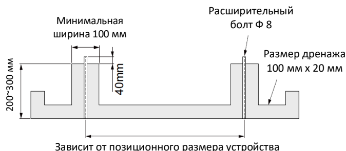
Рисунок 3-2.5. Типовой проект конструкции бетонного основания наружного блока (ед. изм.: мм)
