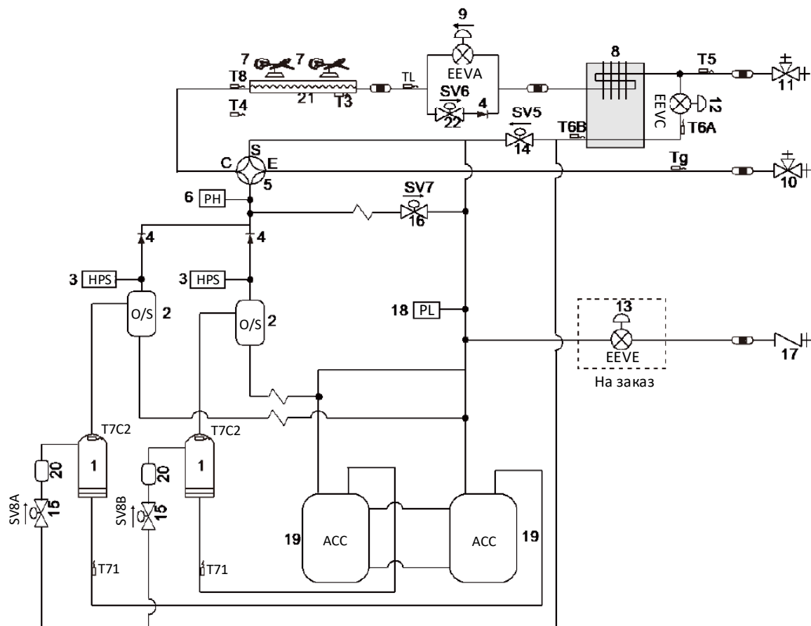
Рисунок 2-4.3. Схема трубопровода модели 28–36 л. с.
