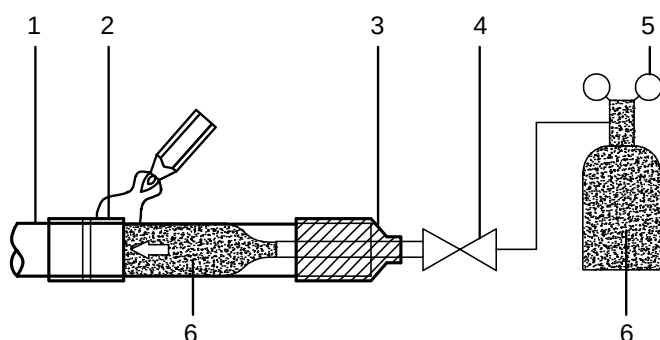
Рисунок 3-5.4. Пропускание азота через трубопровод при пайке
