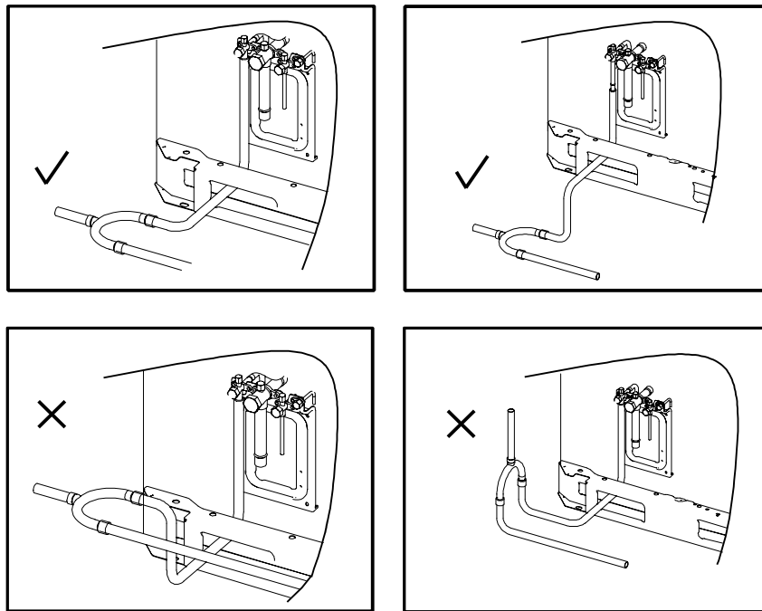
Рисунок 3-5.9. Установка наружных разветвителей
