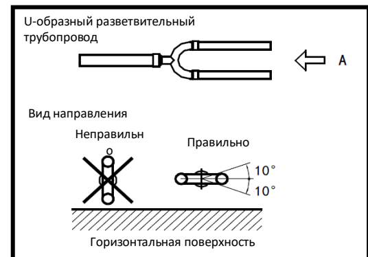
Рисунок 3-5.8. Ориентация разветвителей
