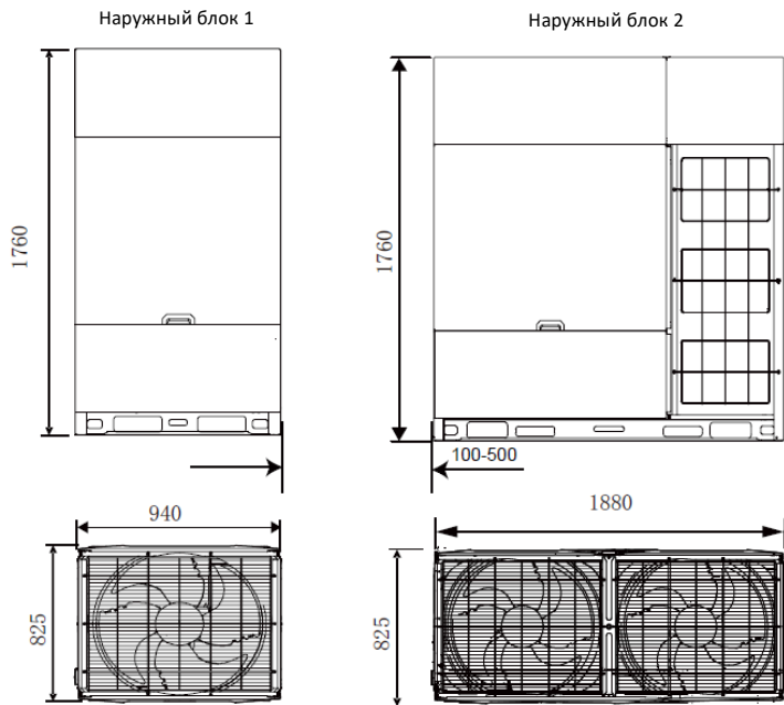
Рисунок 2-2.6. Габариты модели 44 л. с. (ед. изм.: мм)
