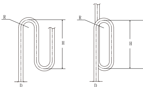
Рисунок 3-4.1. Отвод для возврата масла
