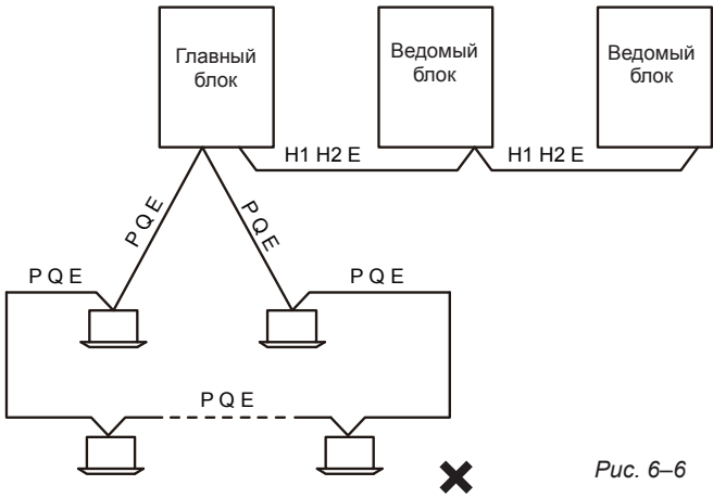
Клеммы связи главного наружного блока
