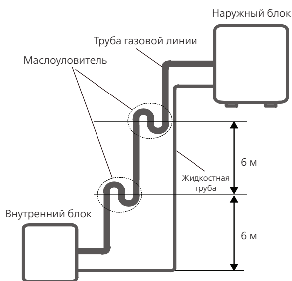
2. Наружный блок установлен выше внутреннего блока
