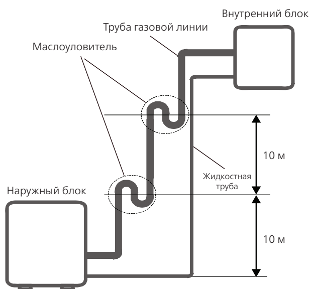
1. Внутренний блок установлен выше наружного блока
