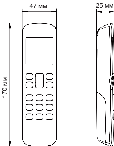
Рисунок 2.1 Размеры пульта ДУ
