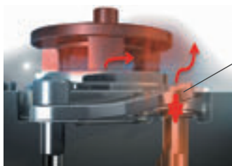
Промежуточный нагнетательный клапан
