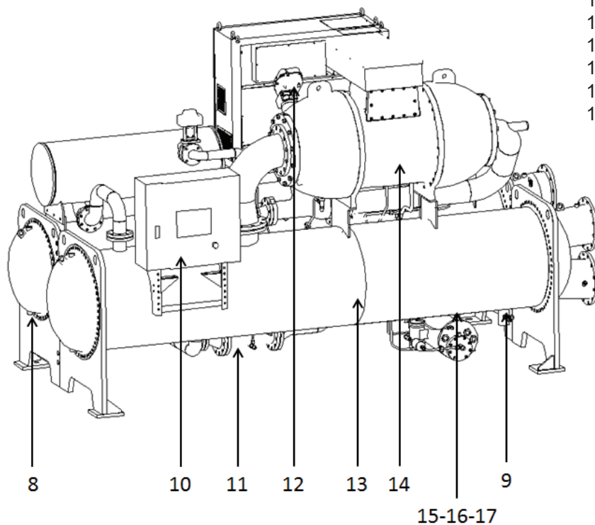
Рисунок 1.3. Схема центробежного чиллера серии с прямым приводом (600RT-1300RT)
