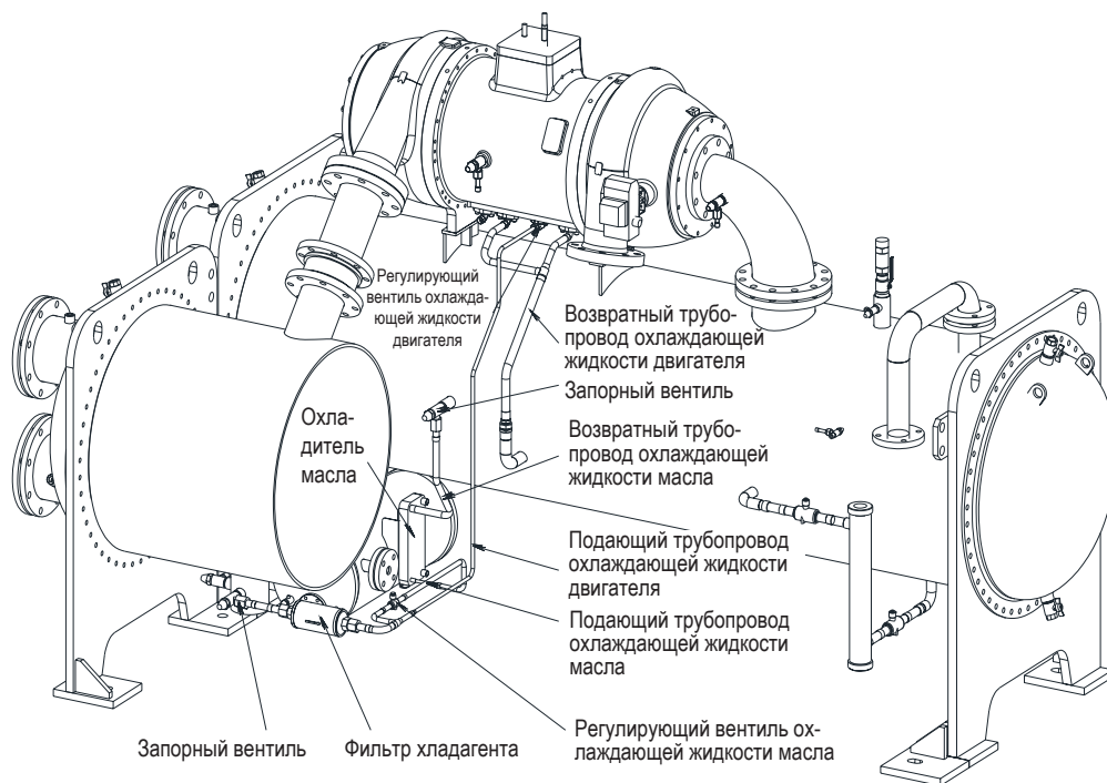
Рисунок 1.6 (а). Охлаждающий трубопровод чиллера серии с прямым приводом (250RT–550RT)
