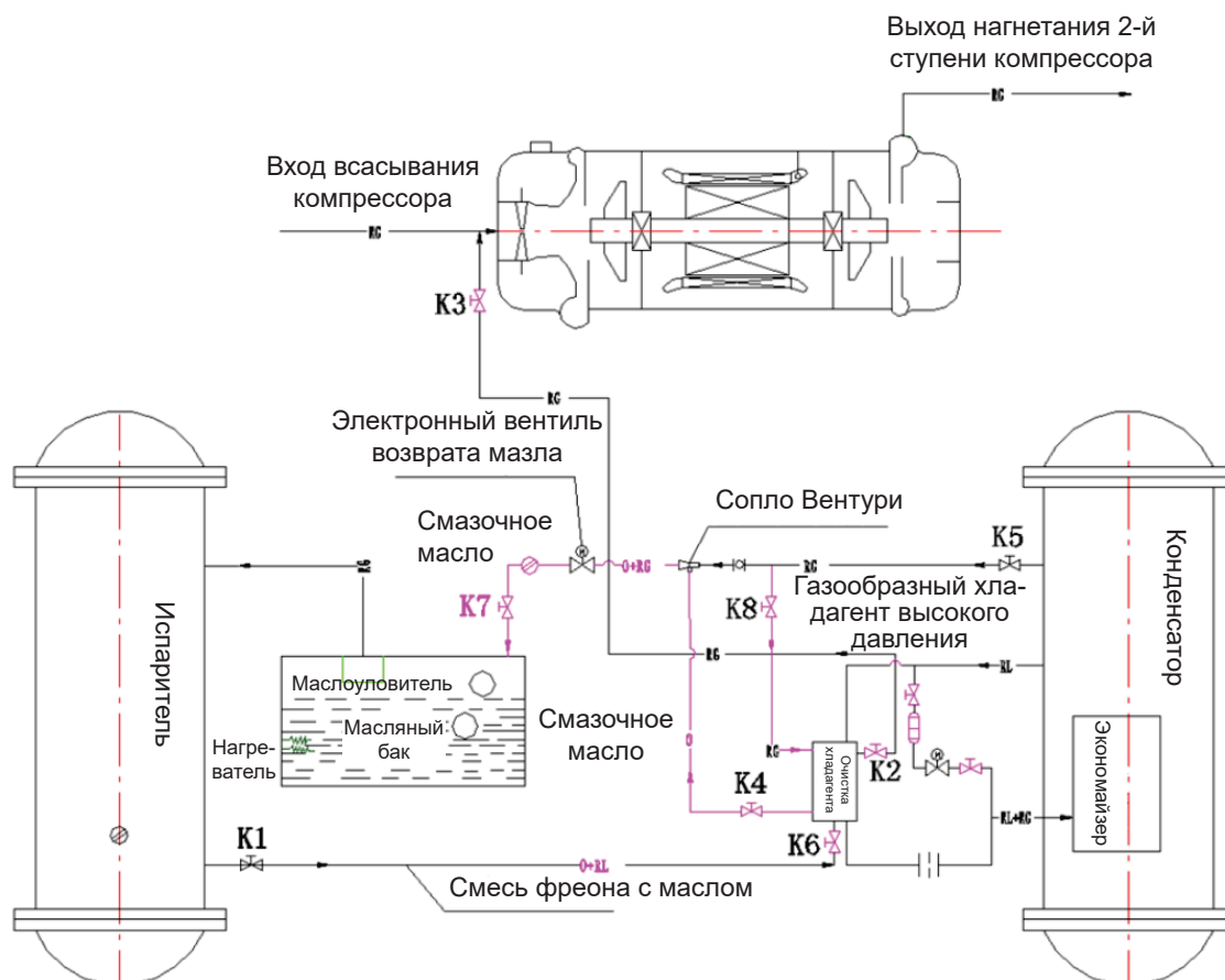
Рисунок 1.8. Схема устройства автоматического извлечения масла чиллера серии с прямым приводом
