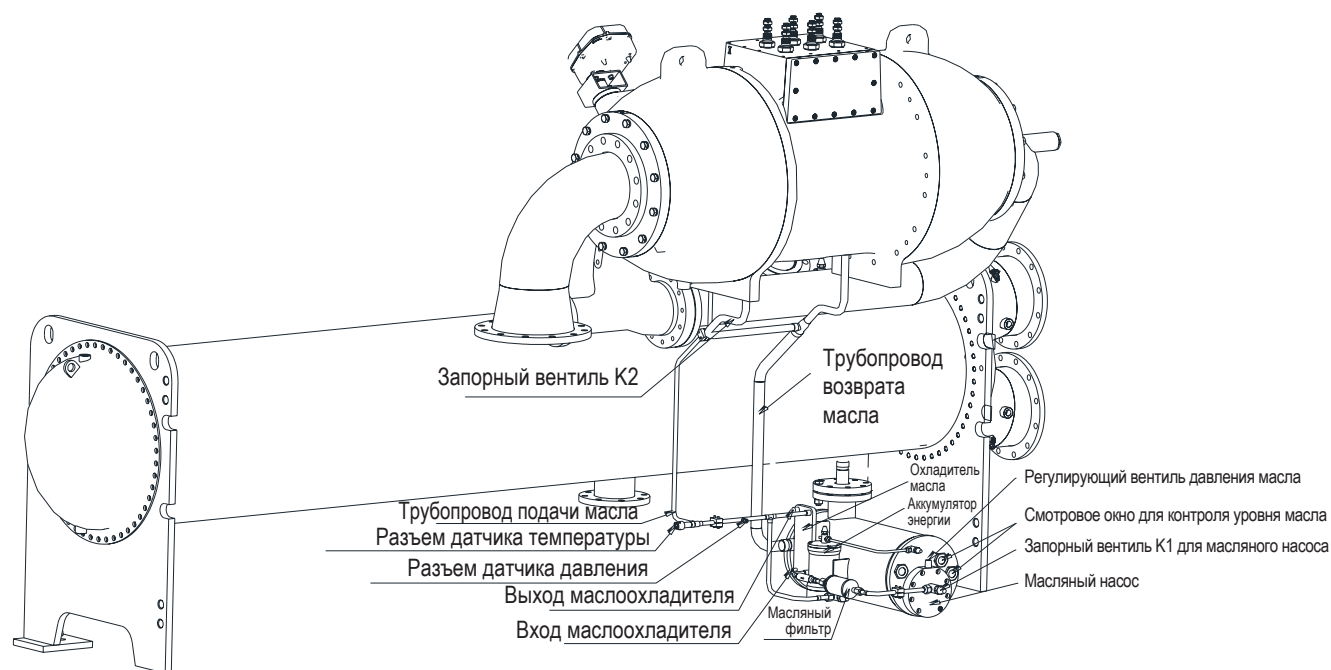
Рисунок 1.4 (b). Схема системы смазки и присоединения трубопроводов чиллера серии с прямым приводом (600RT-1300RT)
