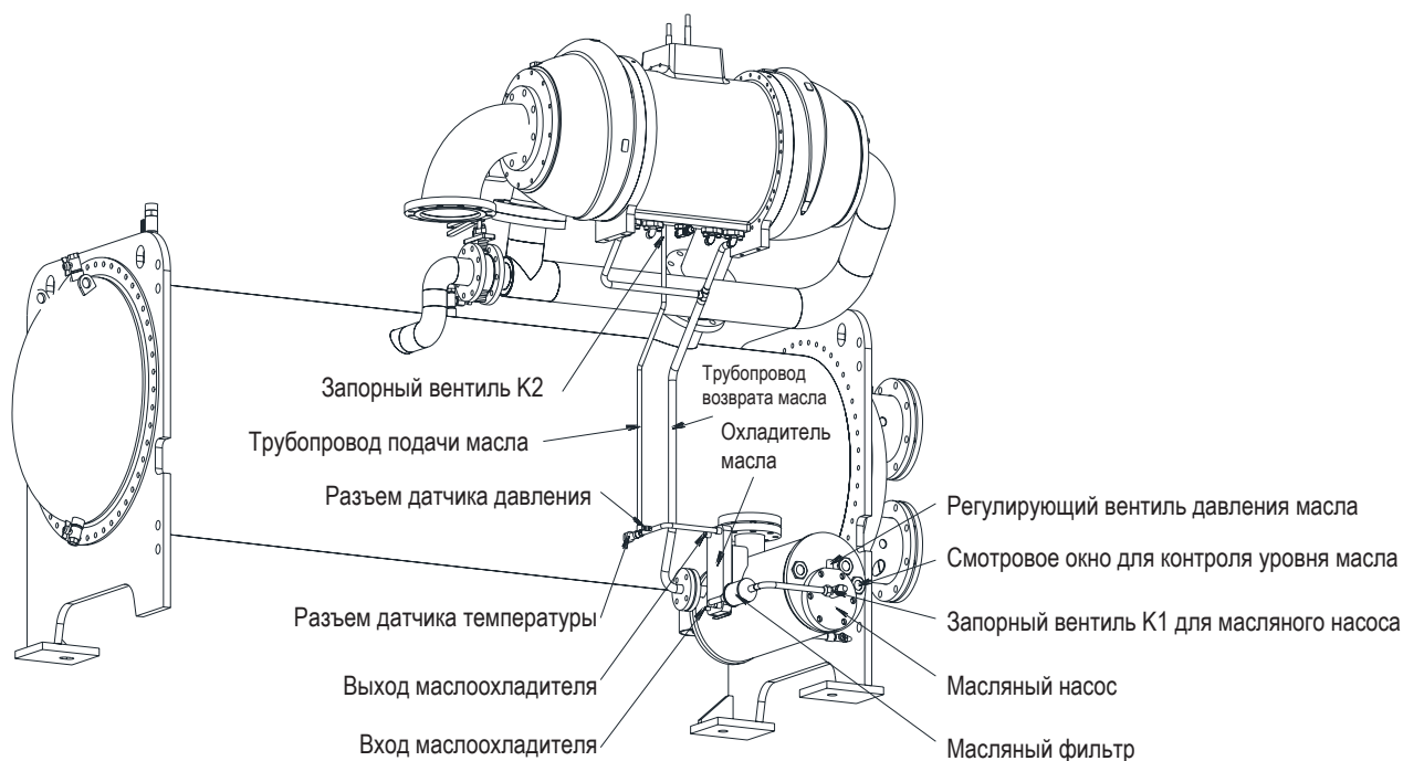
Рисунок 1.4 (а). Схема системы смазки и присоединения трубопроводов чиллера серии с прямым приводом (250RT-550RT)
