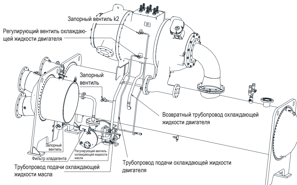
Рисунок 1.6 (b). Охлаждающий трубопровод чиллера серии с прямым приводом (600RT-1300RT)
