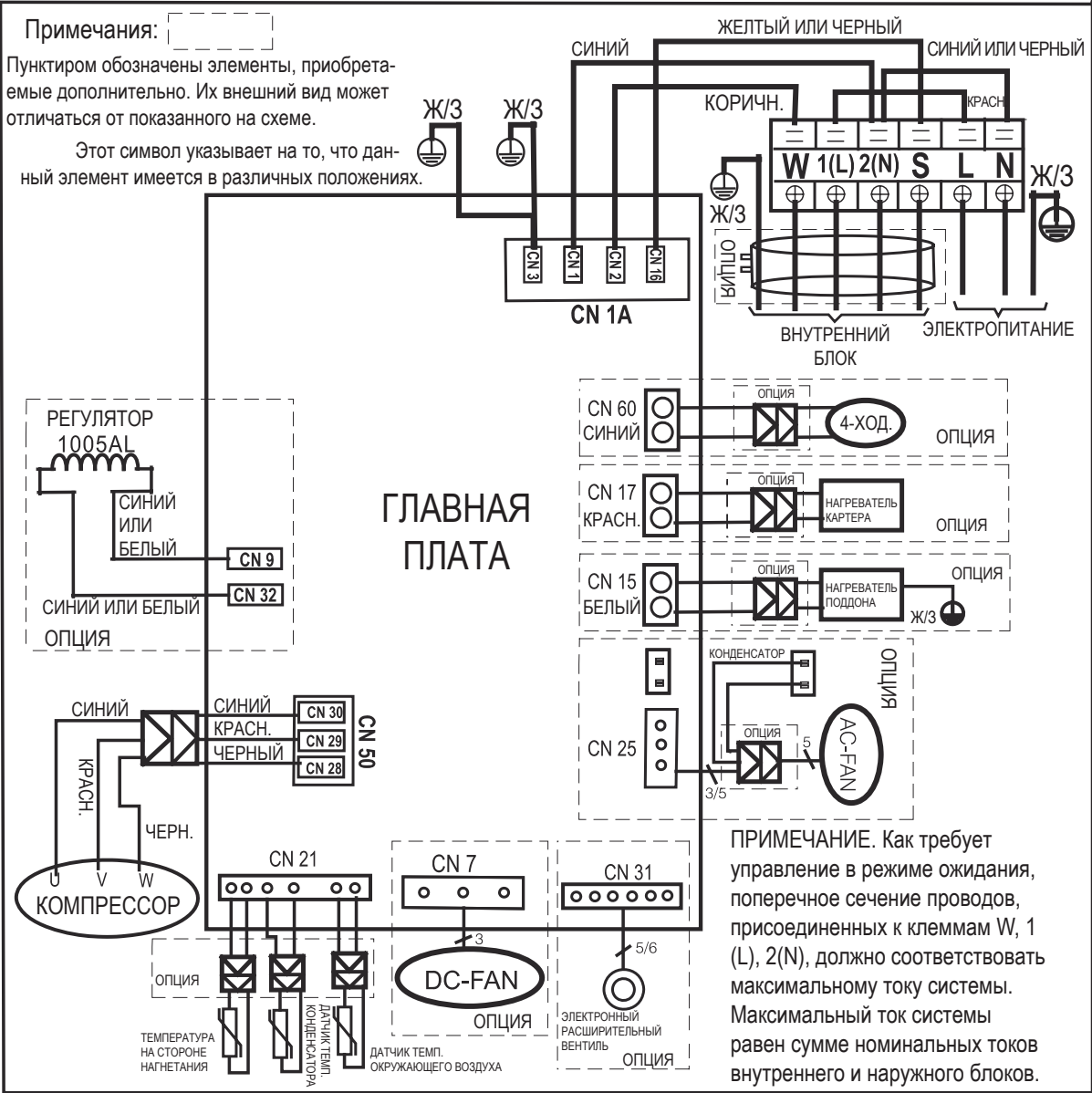
Схема электропроводки наружного блока: 16022000019533
