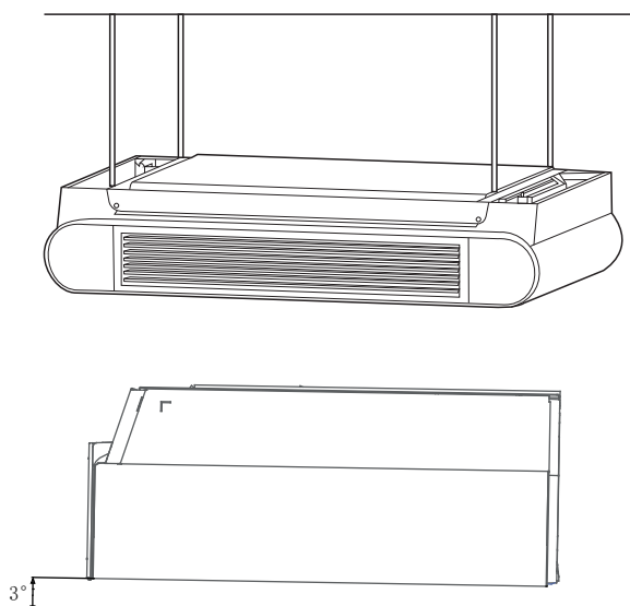
Рисунок 5-5 Схема наружного потолочного монтажа
