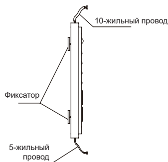
Рисунок 8.2 Плата индикации
