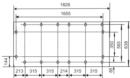
Схема расположения отверстий для заклепок крепления возвратного воздухопровода
