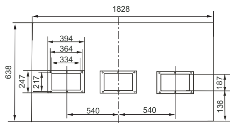
Схема расположения отверстий для болтов крепления воздухопровода воздуховыпускного отверстия MHA-192HWN1
