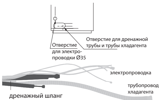
Расположение отверстий для труб/проводов на задней стороне
