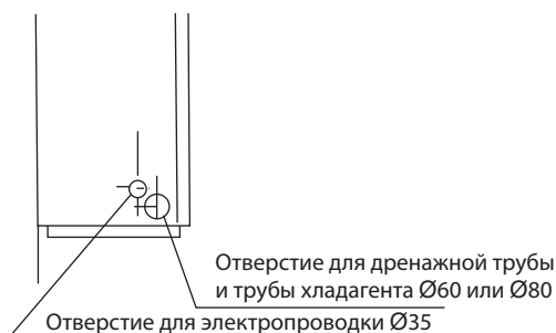
Расположение отверстий для труб/проводов в днище
