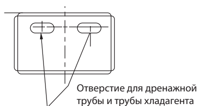
Расположение отверстий для труб/проводов на задней стороне
