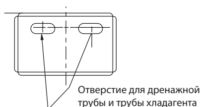
Расположение отверстий для труб/проводов на задней стороне
