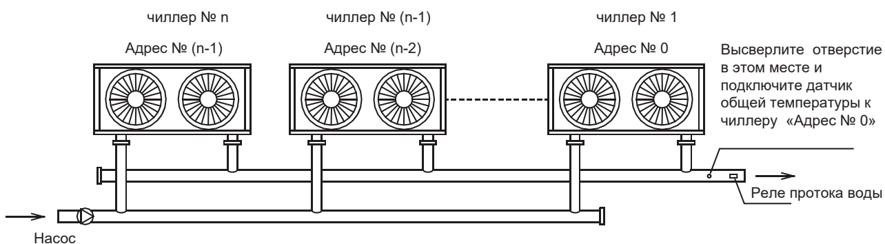
Рис.4-12 (вариант монтажа А - не более 16 чиллеров)
