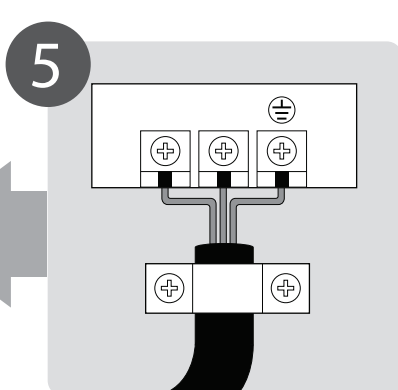
5 Подсоедините кабели
