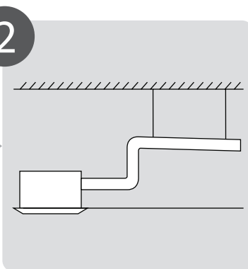
2 Установите дренажную трубу
